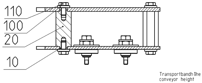
Schnitt/section B-B
