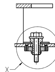
Schnitt/section A-A
