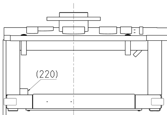
J-J Ansicht B / View B Oben Ansicht / Top View
