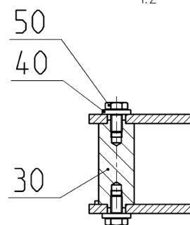
Schnitt/section B-B 1:2
