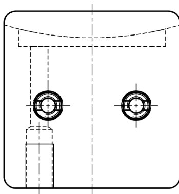
Ansicht B / VIEW B
