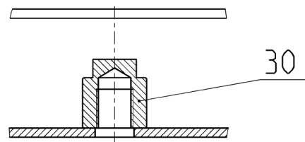
Schnitt/section A-A 1:1
