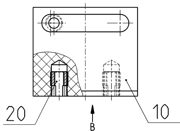
Ansicht B / VIEW B
