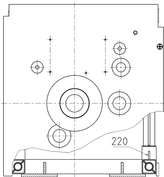
J-J Ansicht B / View B Oben Ansicht / Top View
